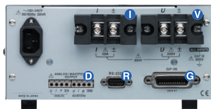
3334-01 背面面板
