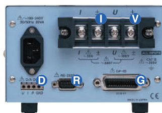
3333-01 背面面板
