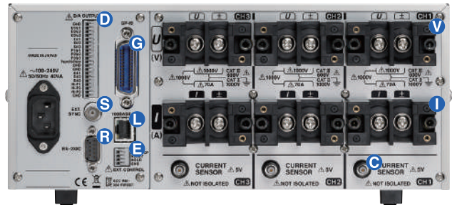
PW3337-03 背面面板
