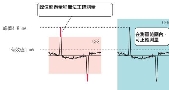
待機時電流波形範例 (CF=峰值/有效值=4.8)
