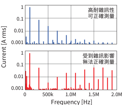
上: CT6904A CMRR 120 dB以上 (100 Hz) 下: CMRR較低的感測器
