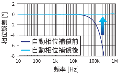
AC/DC電流感測器 CT6904A相位特性補償範例 (代表值)
