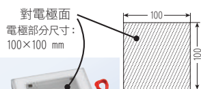
支持台一體型對電極 (SM9001 附件)
