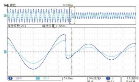
CR模式下:电压幅值、相位、频率突变
