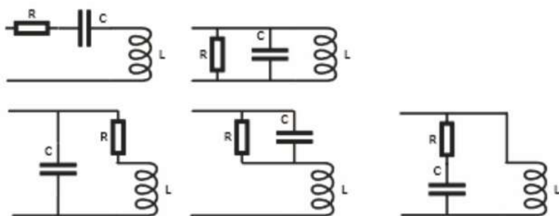
RLC负载网络拓扑图
