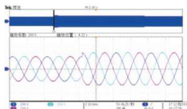
90°高电压穿越
