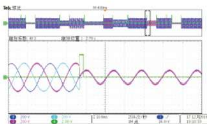
电压相位变化
