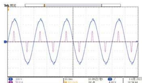
整流型负载-CF=4波形
