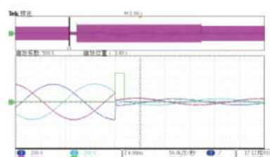
270°高低电压穿越联合测试
