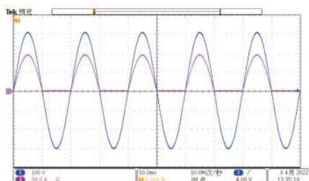
整流性负载-半波整流波形
