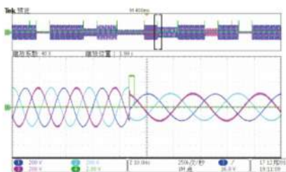
频率电压变化
