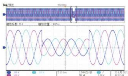
三相相位变化低穿
