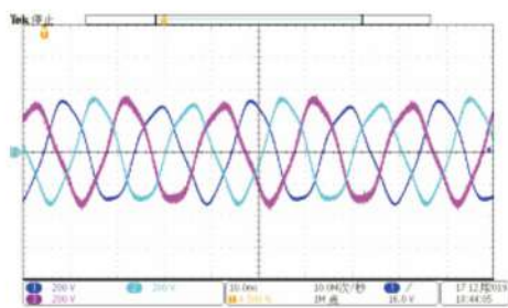
间谐波叠加波形
