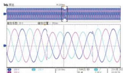
B、C换相低穿
