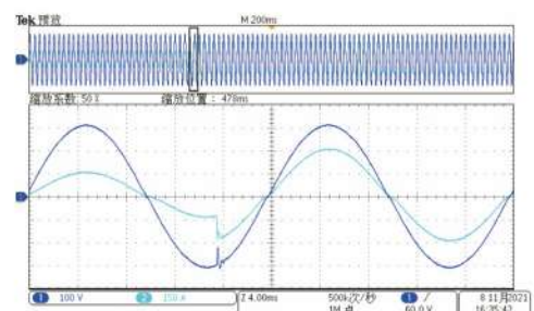
CR模式下:电阻突变
