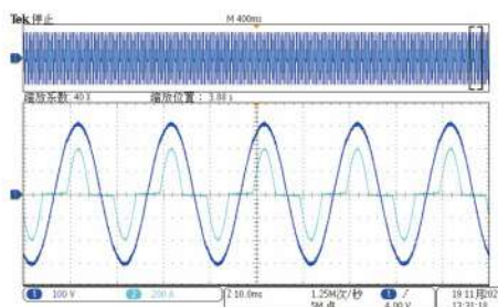
CF=2 CC模式单相电流
