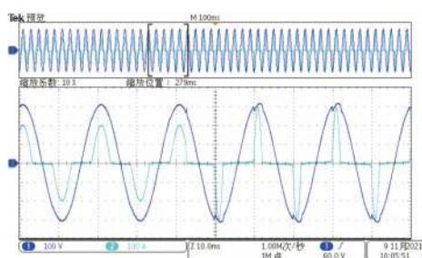
CC模式下:CF突变CF由2变为3
