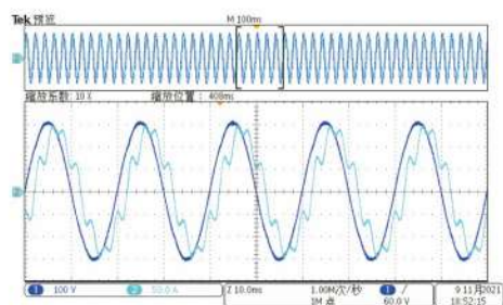
电流谐波模拟
