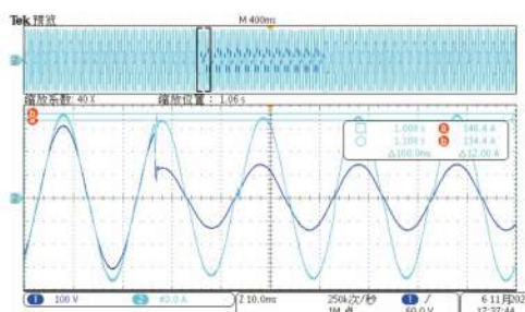
CC模式下:电压幅值变化
