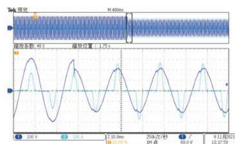
CP模式下:电压幅值突变 CF=2.5
