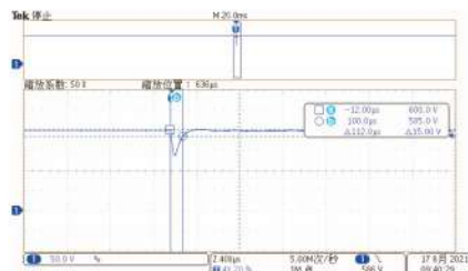
40%-90%负载突加输出电压响应时间
