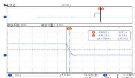
90%~10%负载下降时间
