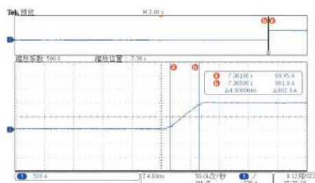
10%~90%负载上升时间
