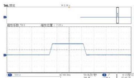
电流缓启动
