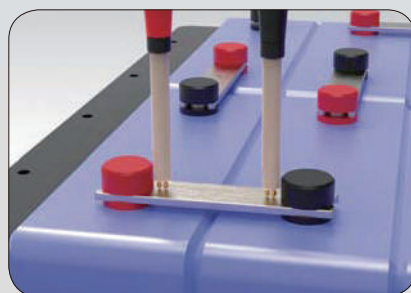
安全量測高壓母線的電阻
