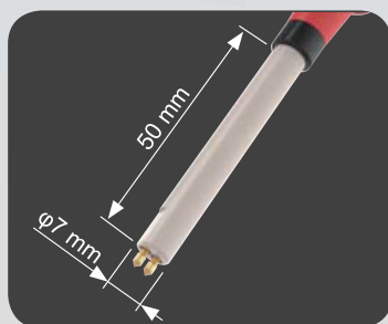
前端長50mm,直徑7mm
