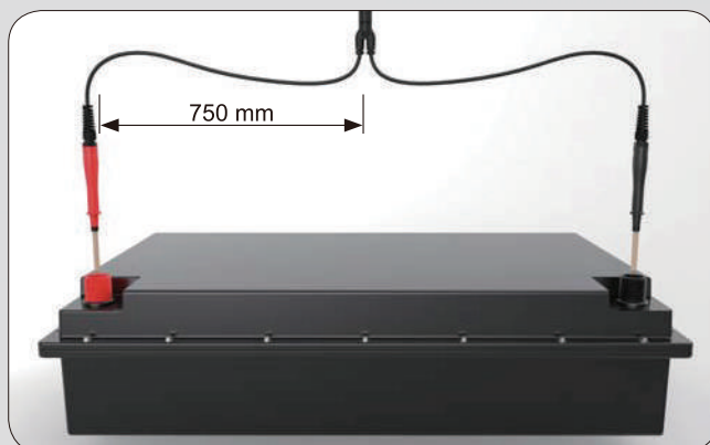
因為測試線加長,對於間距較遠的端子也能測量
