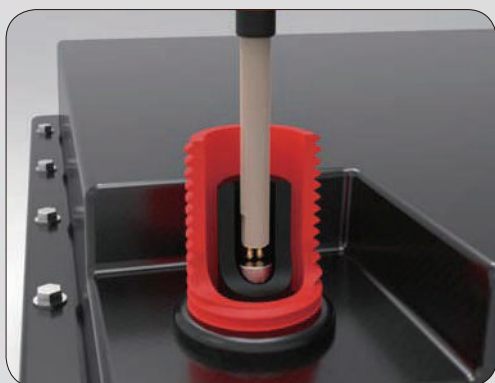
前端加長,深入端子測量也OK (圖為端子部分橫截面示意圖)
